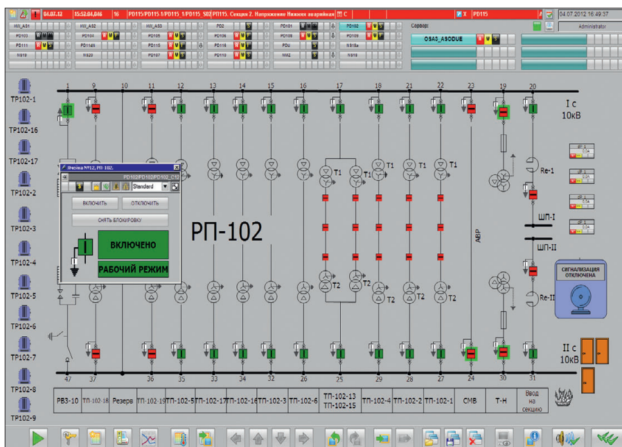
Рис. 5. Мнемосхема РП-102
