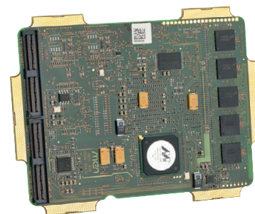
Рис. 4. Вид на КМ формата ESMexpress XM50 со стороны разъёмов
