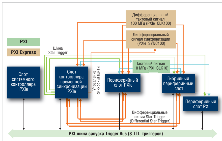
Рис. 2. Шины синхронизации и запуска в PXI Express
