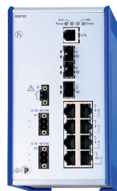
Рис. 3. Коммутатор Ethernet серии RSP компании Hirschmann
