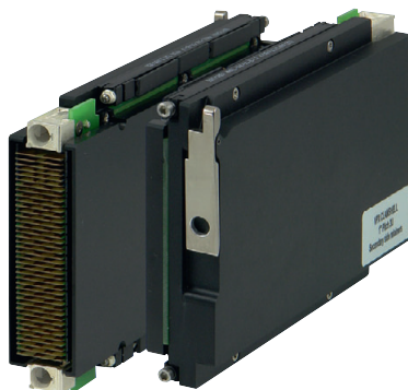
Рис. 6. Два варианта исполнения теплоотводящего кожуха для плат (clamshell) – левый и правый
