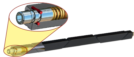
Рис. 11. Клиновой зажим Card-Lock с предохранительным храповым механизмом
