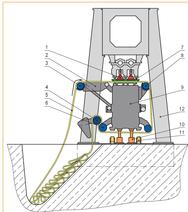
Условные обозначения: 1 — игловый брус; 2 — стол подачи; 3 — тормозной вал; 4 — прижимной вал; 5 — полотно; 6 — тянущий вал; 7 — съёмник; 8 — выпускной вал; 9 — нижний брус; 10 — домкрат; 11 — ролик; 12 — станина.
