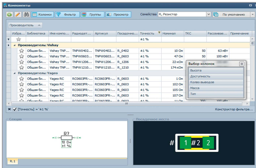
Рис. 3. Поиск компонентов в системе Delta Design
