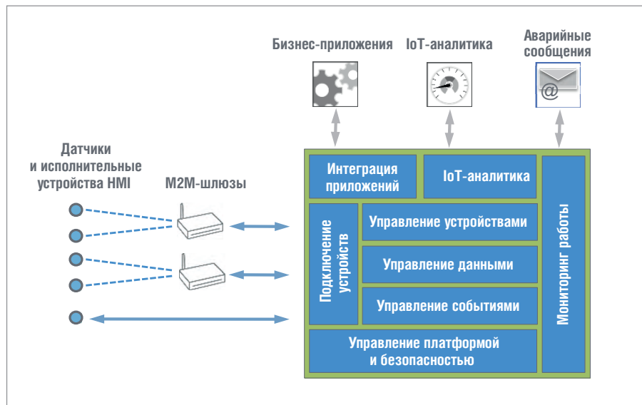
Рис. 5. Структура Everyware Cloud
