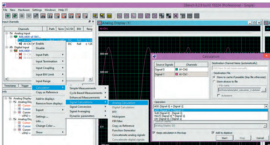
Рис. 48. Настройка типа сигнальной обработки в программе SBench 6 отдельно для каждого входного канала. Для аналоговых вычислений выбран канал AI-Ch0. Диалоговое окно вычислений настроено для добавления сигналов AI-Ch0 и AI-Ch1
