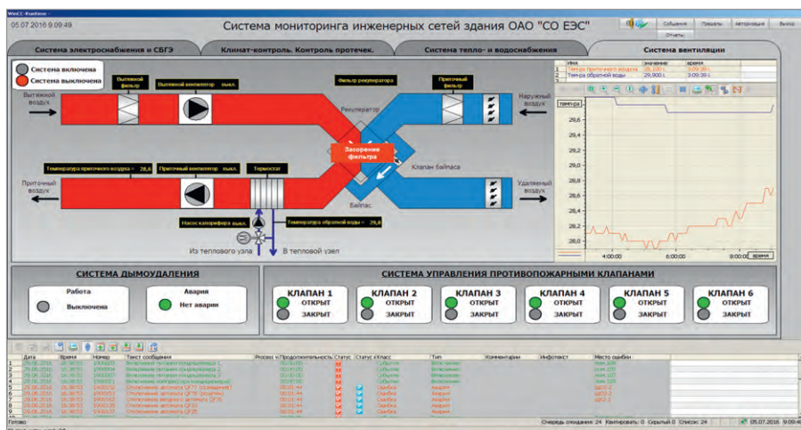
Рис. 9. Экранная форма систем вентиляции и дымоудаления
