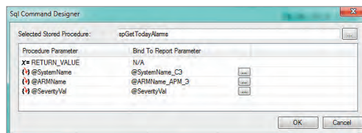
Рис. 8. Окно настройки параметров хранимой процедуры
