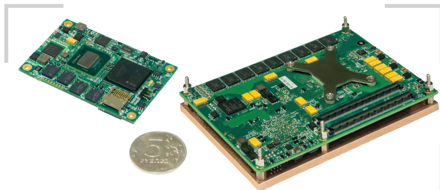
Рис. 2. Примеры SOM-модулей «ДОЛОМАНТ»
