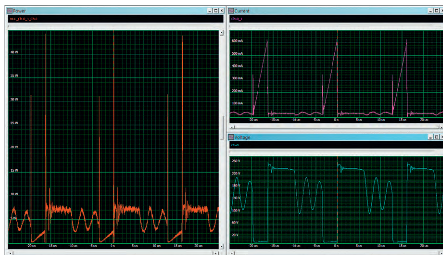
Рис. 50. Использование функции умножения для расчёта мгновенной мощности от волновых форм тока и напряжения в импульсном блоке питания
