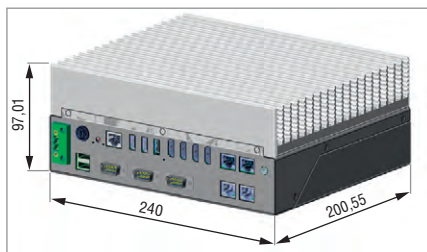
Рис. 2. Прототип изделия
