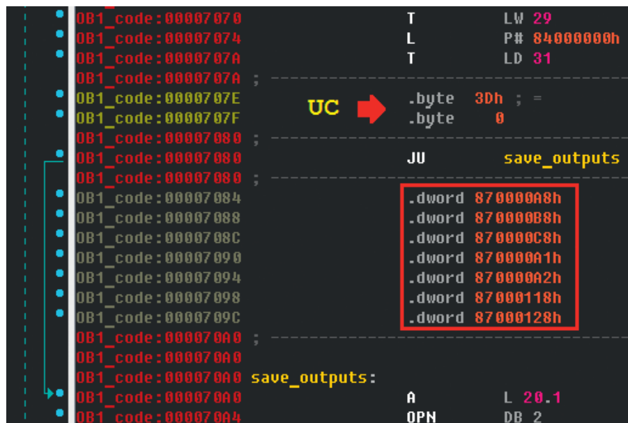
Рис. 3. Передача параметров в AG_RECV
