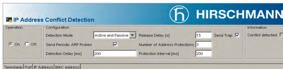
Рис. 6. Настройка механизма обнаружения конфликта IP-адресов
