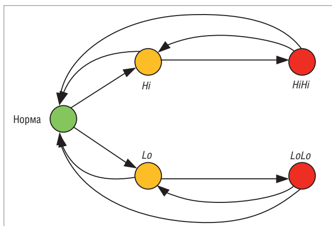
Рис. 2. Диаграмма изменения состояний аналогового аварийного сигнала
