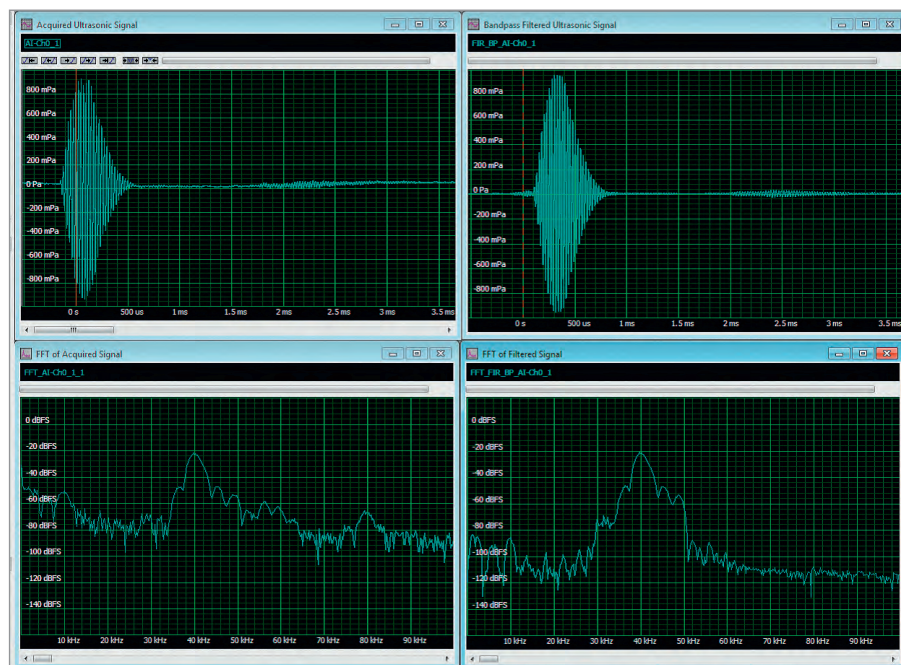
Рис. 56. Результаты применения полосового FIR-фильтра с частотами отсечки от 30 до 50 кГц для ультразвукового сигнала частотой 40 кГц. Исходный сигнал и его FFT находятся в левой части экрана. Справа отображается отфильтрованный сигнал и его FFT. Выравнивание в отфильтрованной базовой линии получено в результате устранения низкочастотной составляющей
