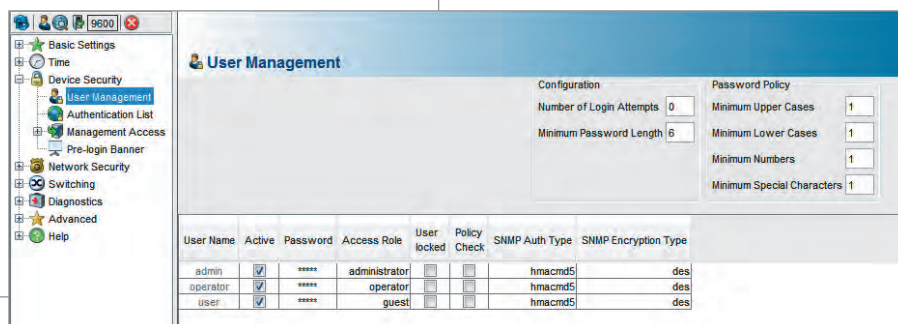
Рис. 3. Страница настроек коммутатора с распределением уровня доступа
