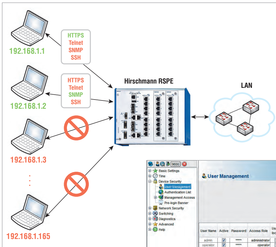
Рис. 2. Визуальное представление правил безопасности
