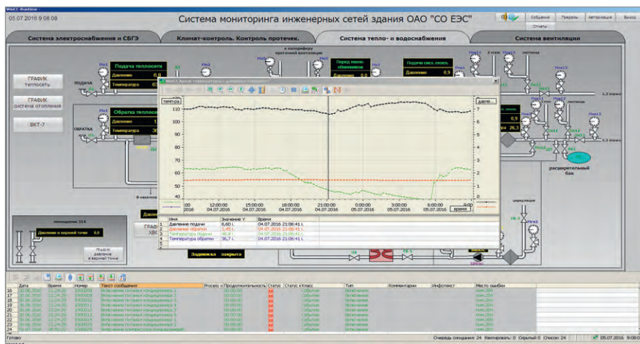
Рис. 8. Экранная форма системы тепло- и водоснабжения с всплывающим окном графиков температур и давлений
