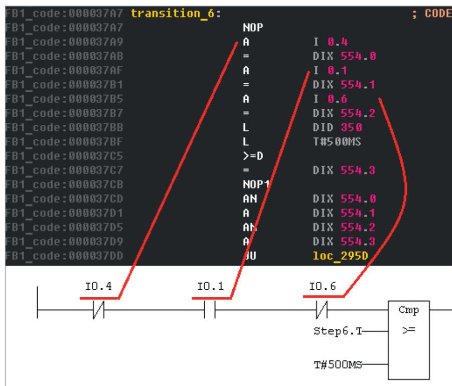
Рис. 5. Соответствие LAD-кода перехода № 6 МС-коду
