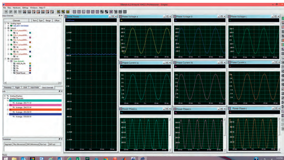
Рис. 61. Расчёт фазовой мощности с использованием значений всех трёх фазовых напряжений и токов в простом примере
