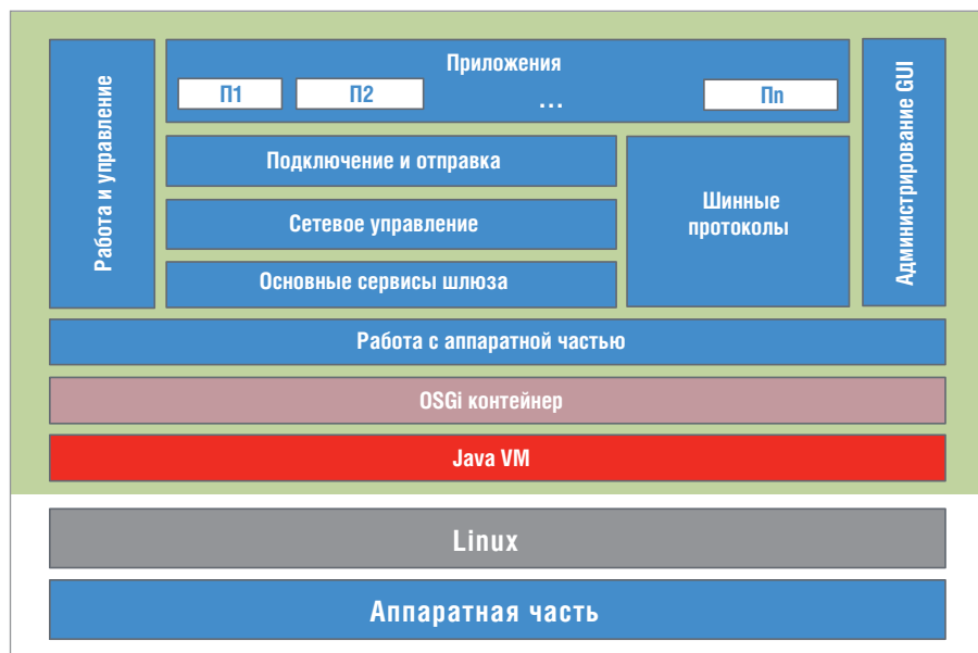
Рис. 3. Структура Everware Software Framework
