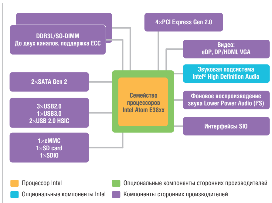
Рис. 2. Блок-схема для семейства процессоров Intel® Atom™ E38xx [2]
