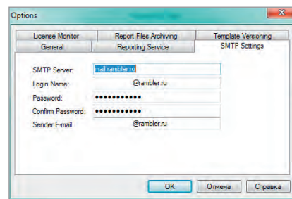
Рис. 15. SMTP-настройки ReportWorX
