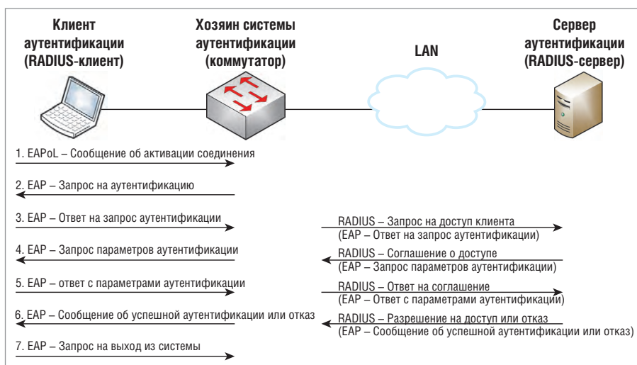
Рис. 5. Аутентификация пользователей в соответствии с 802.1x, протокол RADIUS
