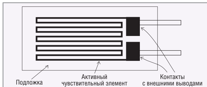
Рис. 2. Структура металлического тензодатчика
