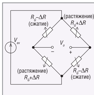
Рис. 7. Использование четырёх тензодатчиков для повышения чувствительности схемы измерения и компенсации температурной погрешности,
