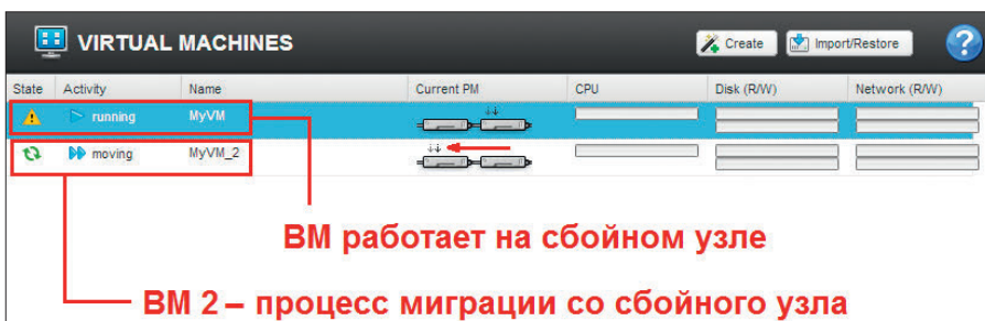
Рис. 4. Перенос приложений
