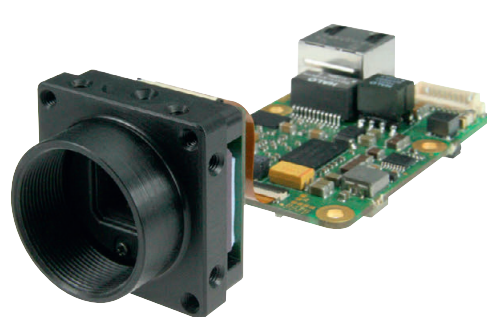
Рис. 5. Встраиваемая камера серии Giganetix Board Level
