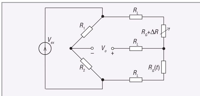
Рис. 11. Подсоединение тензодатчика с внутренним
