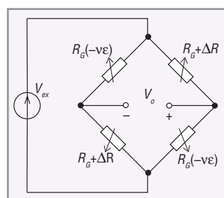
Рис. 9. Схема с четырьмя тензодатчиками, но с отличающимся от представленного на рис. 8 размещения датчиков в плечах моста,
