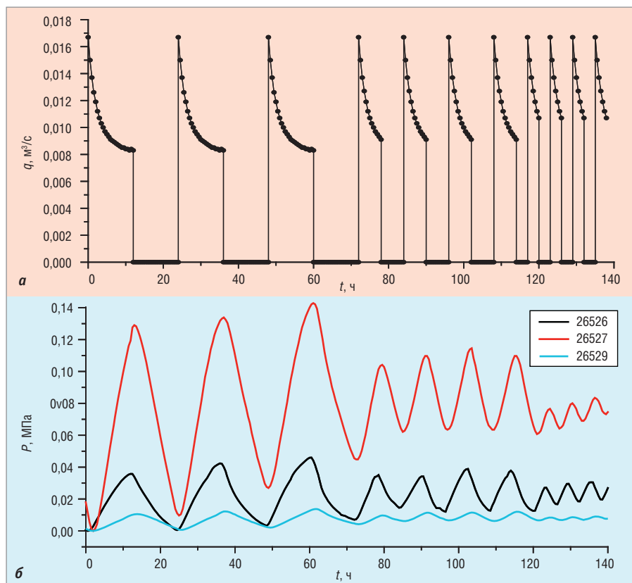
Рис. 2. Периодические колебания дебита ( q , м³/с), задаваемые с периодами 24, 12 и 6 часов на возмущающей скважине (а), и изменения давлений ( P , МПа) на скважинах-приёмниках (б) [4]
