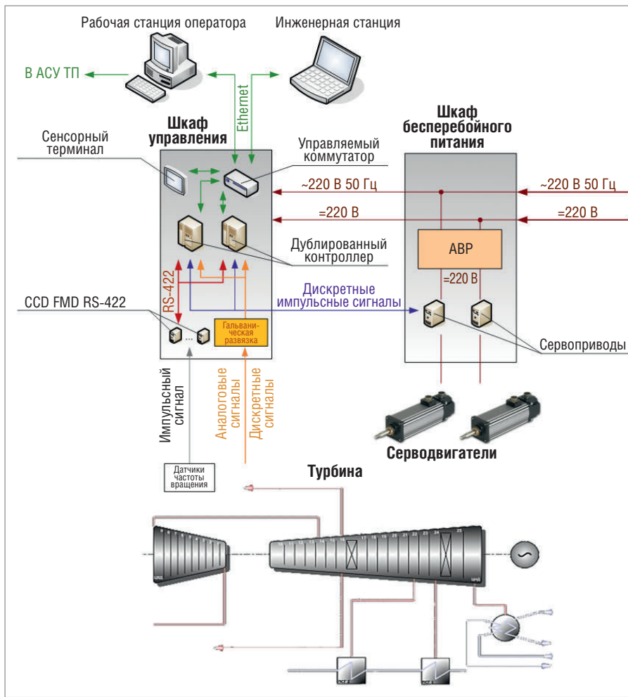
Рис. 1. Структура ЭЧСРиЗ в общем виде
