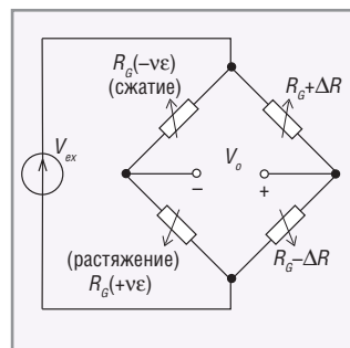
Рис. 8. Схема с четырьмя тензодатчиками, два из которых расположены перпендикулярно направлению силы, \varepsilon = \frac{-2 \cdot V_\gamma}{GF \cdot (v+1)}
