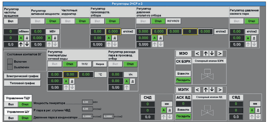
Рис. 4. Внешний вид экрана «Регулирование» (основной управляющий экран)
