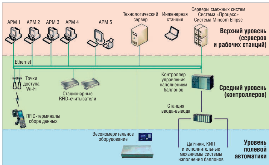
Рис. 5. Архитектура системы
